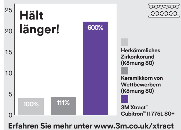
Standzeit (min)
